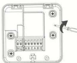
Fixati capacul de pe spatele receptorului de perete cu 4 suruburi furnizate
