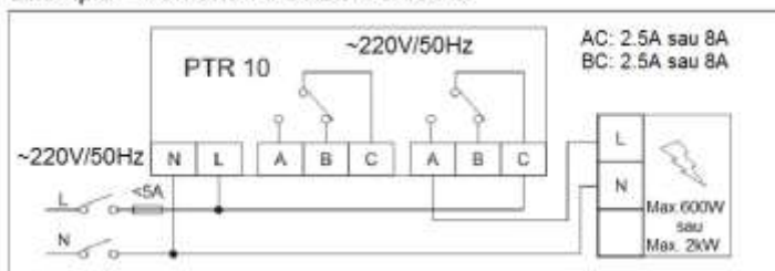
Exemplu – comanda incalzitor electric
