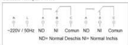
Contacte Receptor PTR10
