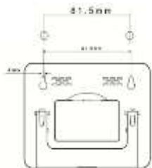
Pozarea pe perete
