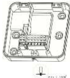
Insurubiti cablurile electrice cu papuci metalici cu diametru de max 2.5mm 2 , conform schemei electrice utilizate
